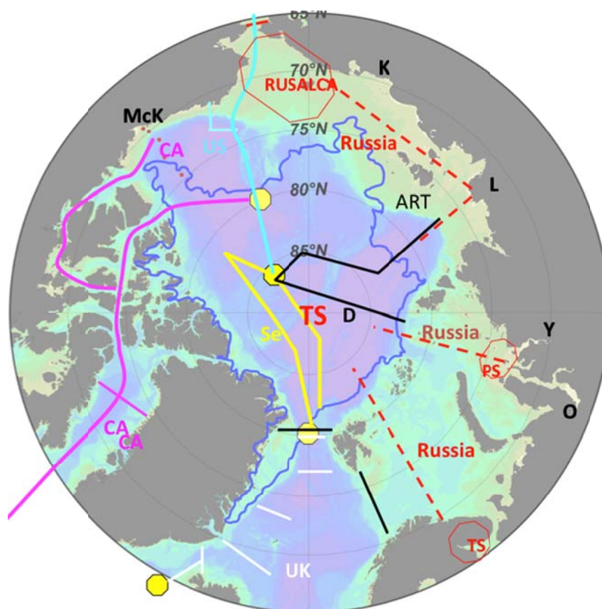
Рисунок. Схематическое положение потенциальных российских океанологических разрезов (красные пунктирные линии) в Северном Ледовитом океане, запланированных в рамках программы GEOTRACES в 2012 году. Положение разрезов других стран-участников программы показано сплошными линиями: CA – Канада, фиолетовым цветом; D – Германия, черным цветом; Se – Швеция, желтым цветом [1 st Russian GEOTRACES Workshop: Final Statement, 2012].
